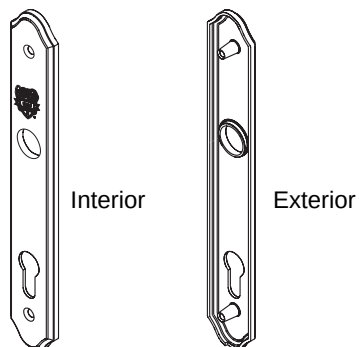
#14 & 20) Active Handleset Escutcheon Plates Style 1
